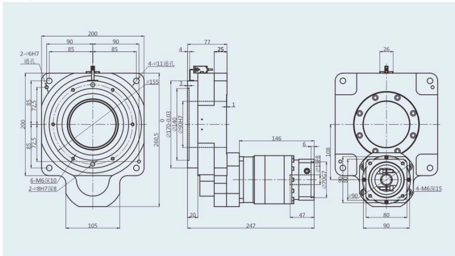
HRTZ200-L2 配750伺服接口 for 750W Servo Interface
