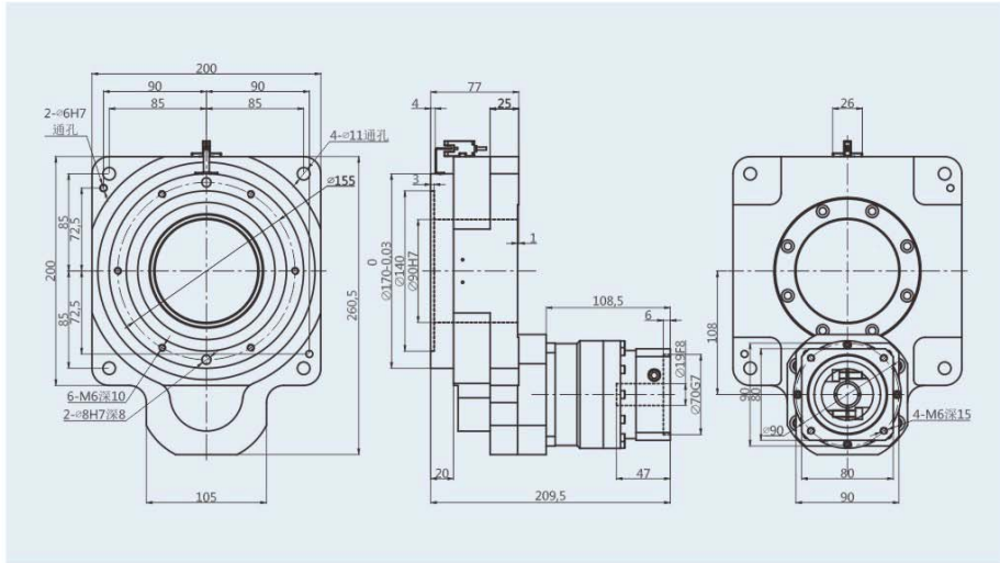
HRTZ200-L1 配750伺服接口 for 750W Servo Interface
