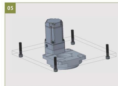
吊装 Hoisting
