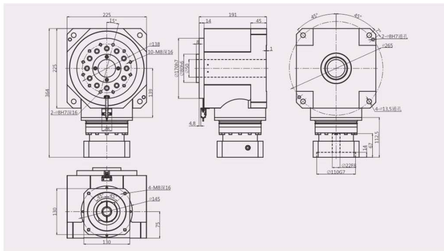
HRMD225-L1 配1KW伺服接口 for 1KW Servo Interface
