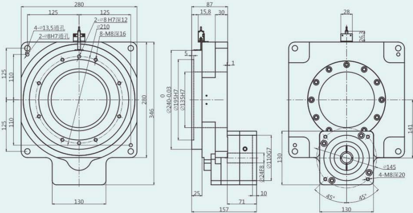
HRTJ280-10 配1KW伺服接口 for 1KW Servo Interface
