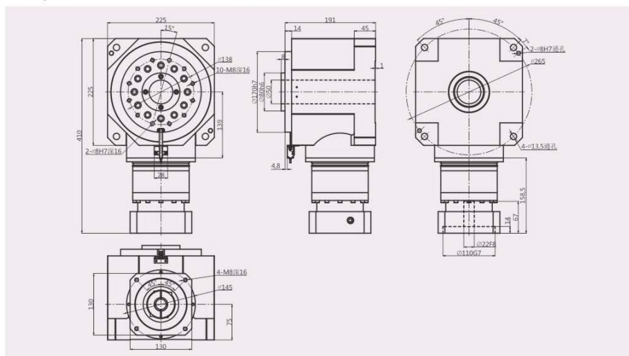
HRMD225-L2 配1KW伺服接口 for 1KW Servo Interface
