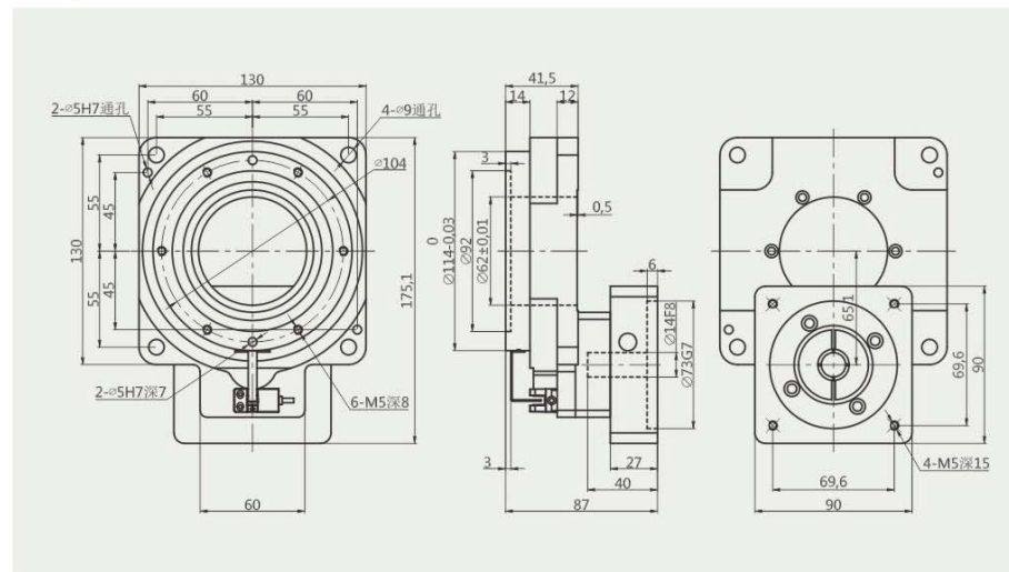
HRT130-10 (18) 配86步进接口 for 86 Stepper Interface
