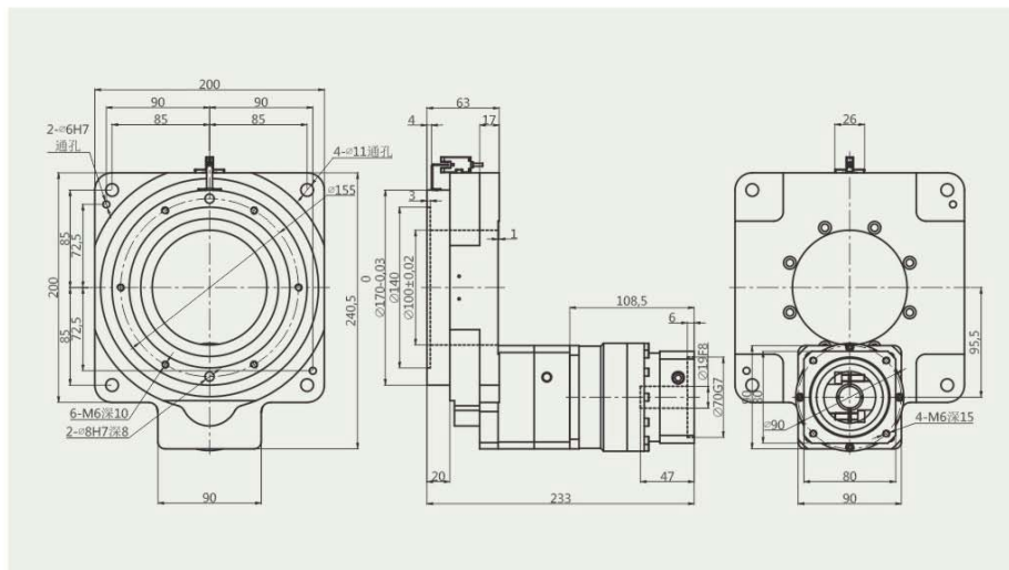
HRT200JS-30 配750W伺服接口 for 750W Servo Interface
