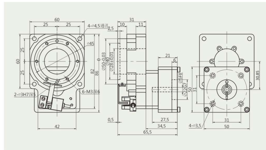
HRT62-10 配42步进接口 for 42 Stepper Interface
