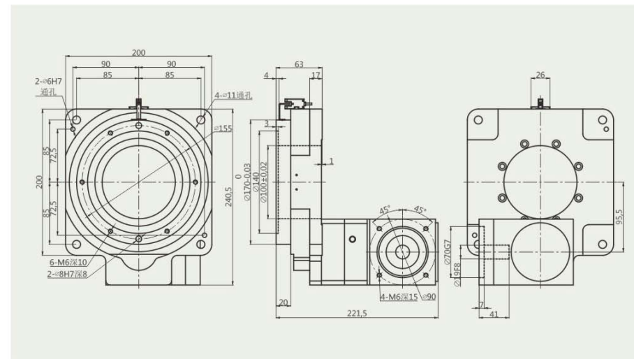
HRT200RY-10 配750W伺服接口 for 750W Servo Interface
