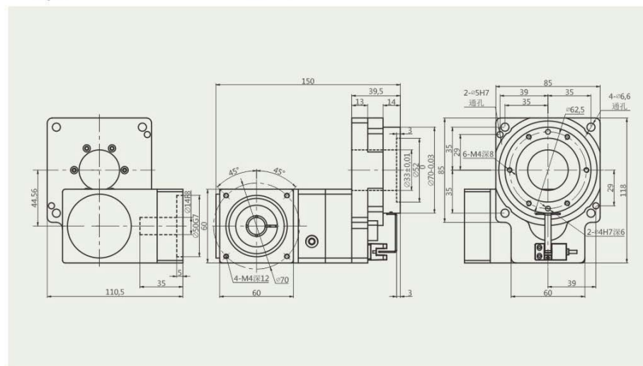
HRT85RZ-5 配400W伺服接口 for 400W Servo Interface
