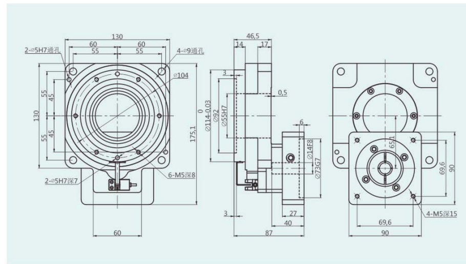
外形尺寸图表 Outline dimensional
