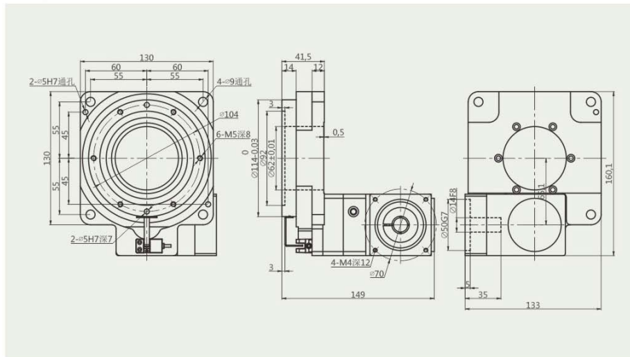
HRT130RY-10 配400W伺服接口 for 400W Servo Interface
