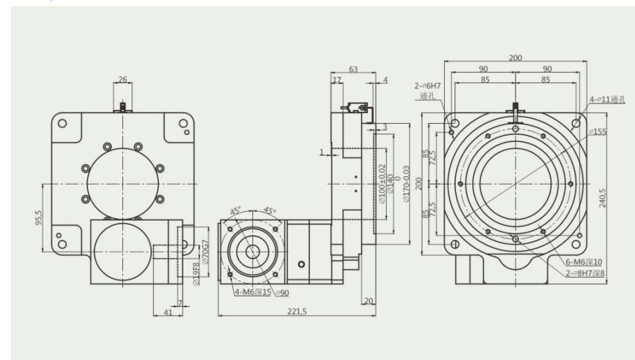
HRT200RZ-10 配750W伺服接口 for 750W Servo Interface
